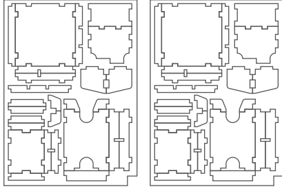
Sheet A1
